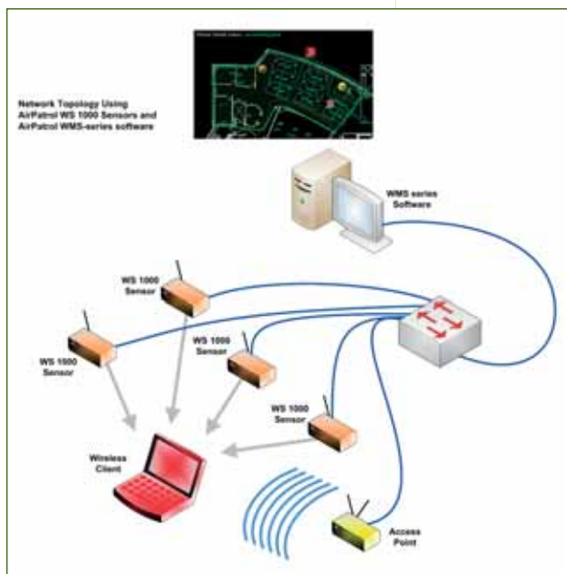
Σχήμα 1. Τοπολογία Διασύνδεσης
